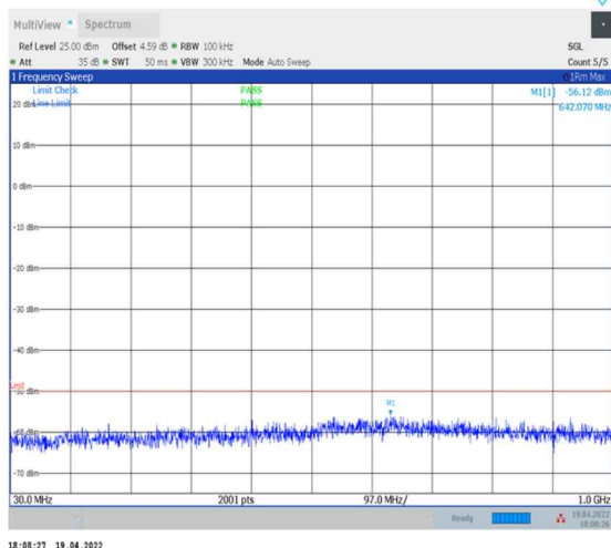
1-N30--15-10-L-1-DFT-PI2BPSK-Inner_1RB_Left- 1@1-30-1000-Ant0--56.12--50-PASS
