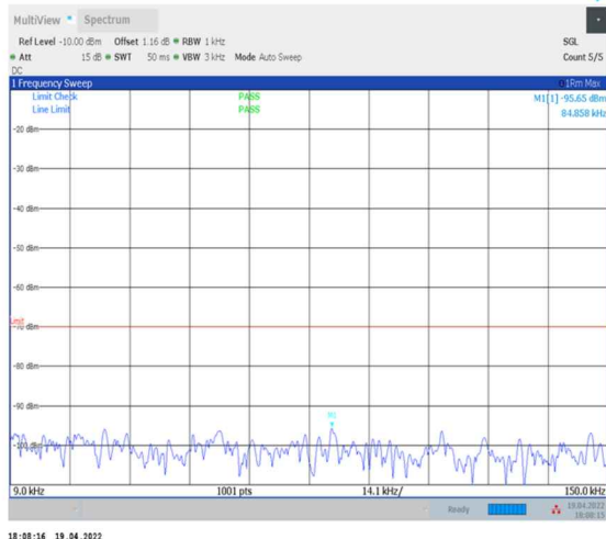
1-N30--15-10-L-1-DFT-PI2BPSK-Inner_1RB_Left- 1@1-0.009-0.15-Ant0--95.65--70-PASS
