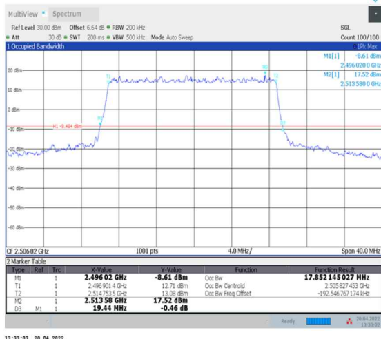
1-N41--30-20-L-1-DFT-QPSK-Outet_Full-50@0-Ant0-17.852-19.440-≤20-PASS
