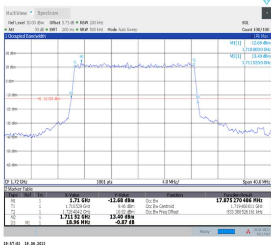
1-N66-PC3-15-20-L-2-DFT-PI2BPSK-Outer_Full-100@0-Ant0-17.875-18.960-≤20-PASS
