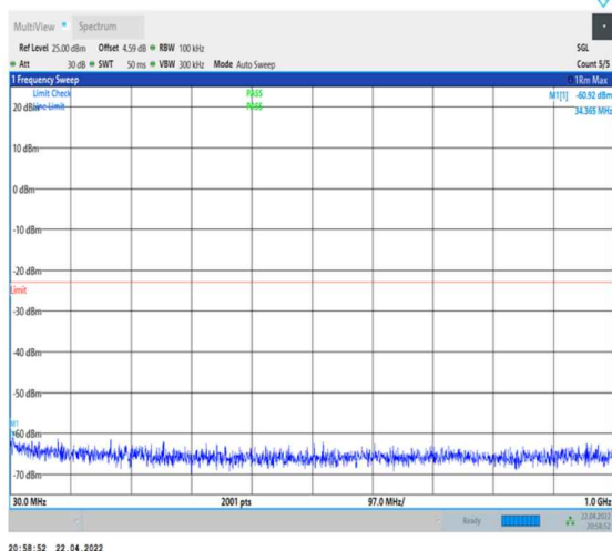
1-N66-PC3-15-40-L-1-DFT-PI2BPSK- Inner_1RB_Left-1@1-30-1000-Ant0--60.92--23- PASS
