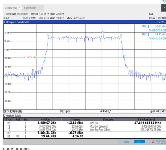
1-N78-3450-3550--30-20-L-2-DFT-PI2BPSK-Outer_Full-50@0-Ant0-17.85-19.440-≤20-PASS
