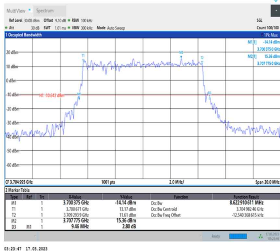
1-N78-3700-3800-PC1-30-10-L-3-DFT-16QAM-Outer_Full-24@0-Ant0-8.623-9.460-≤10-PASS
