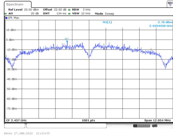
MIMO Ant. 8
