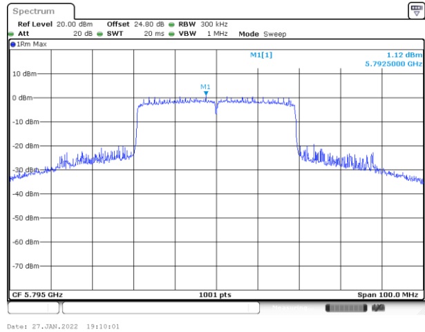
MIMO Ant. 8
