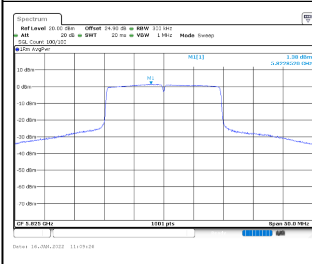
MIMO Ant. 9
