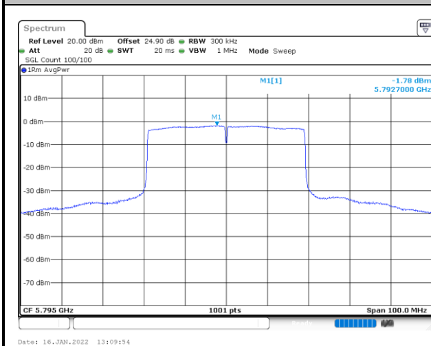
MIMO Ant. 9
