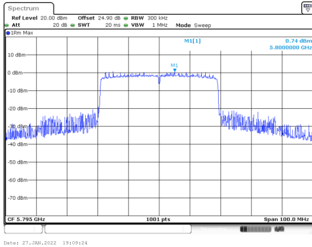
MIMO Ant. 9
