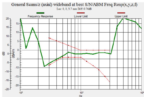
Fig. 8.7 CDMA2000 BC1 Ch600
