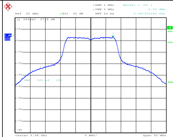
802.11a CH116 5580MHz
