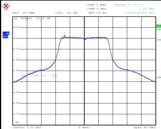
802.11a CH100 5500MHz
