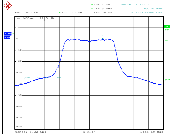
802.11a CH64 5320MHz
