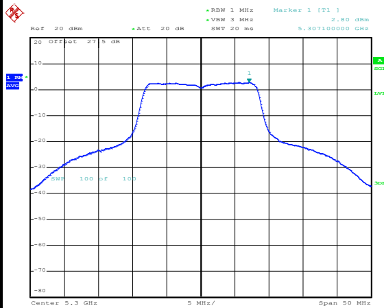
802.11a CH60 5300MHz
