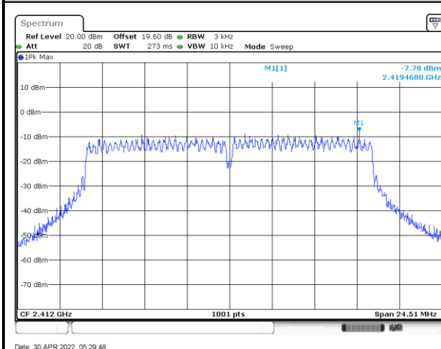
MIMO Ant. 9
