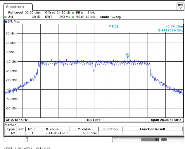
MIMO Ant. 2
