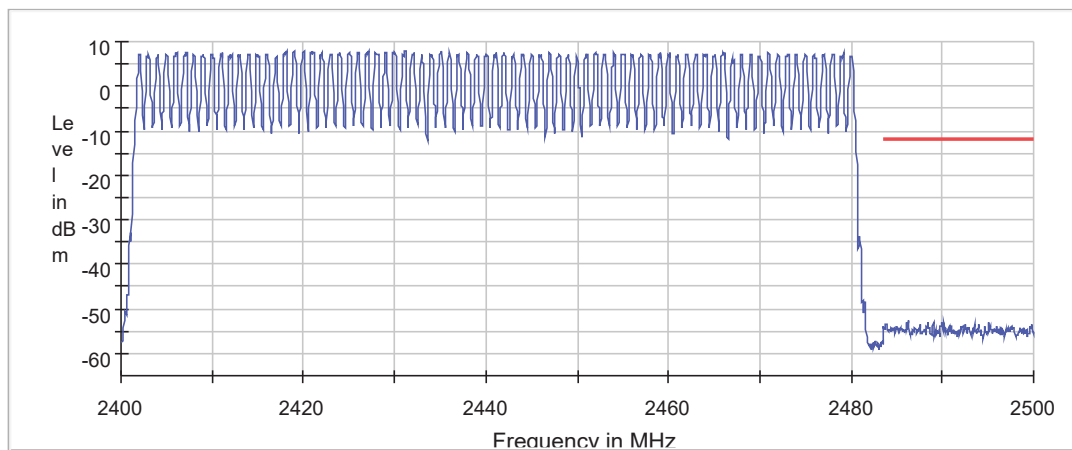
Band Edge
