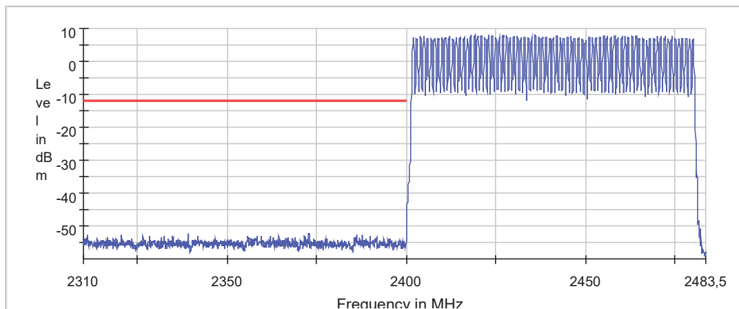
Band Edge
