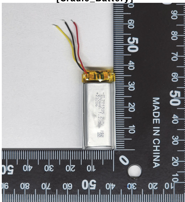
[Cradle_Battery]
