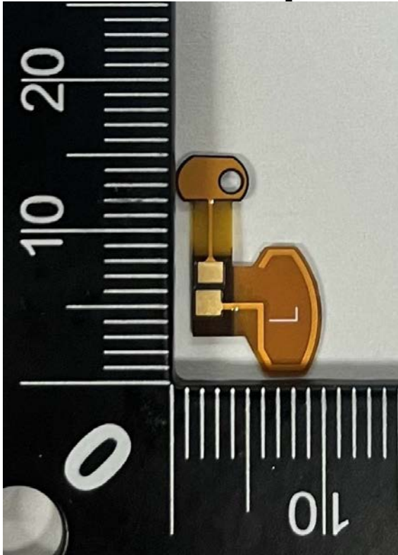
[Earbud_Right_Antenna]
