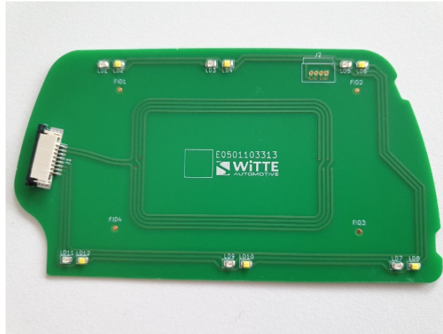
flinkey BLE Keybed PCB top side
