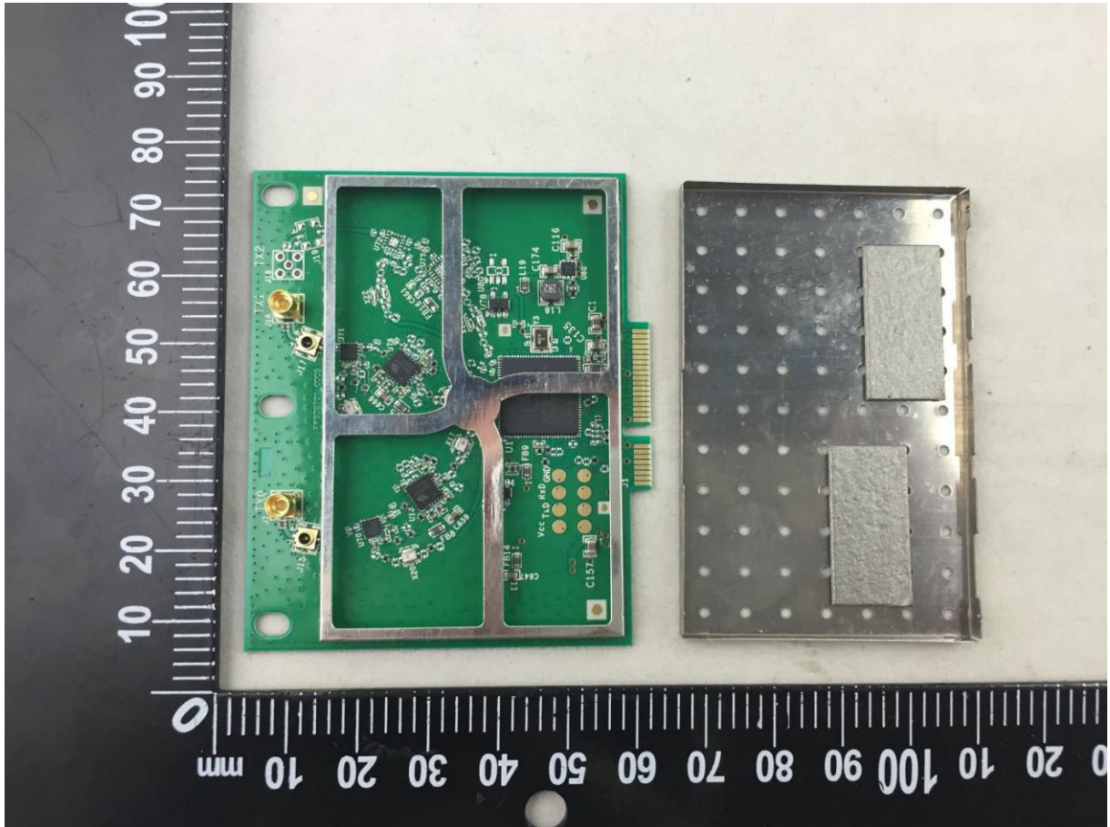
EUT UNCOVER
