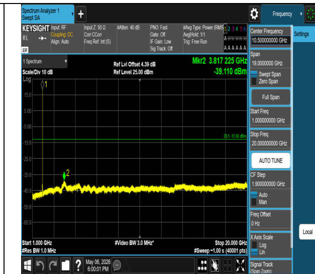
Band II-9400-1000~20000MHz-PASS
