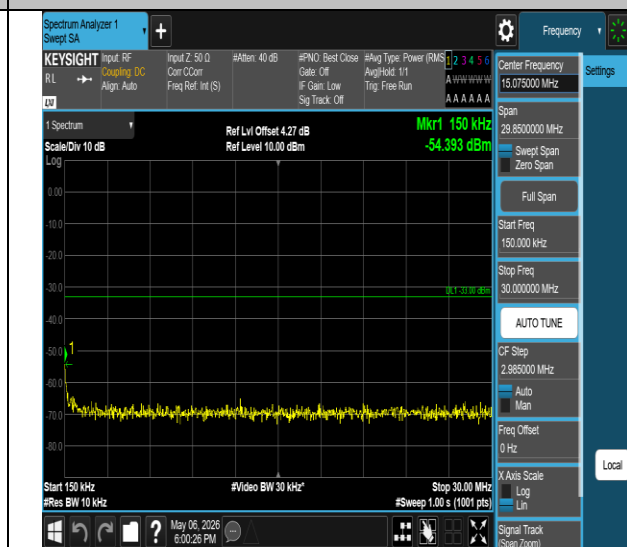
Band II-9538-0.15~30MHz-PASS
