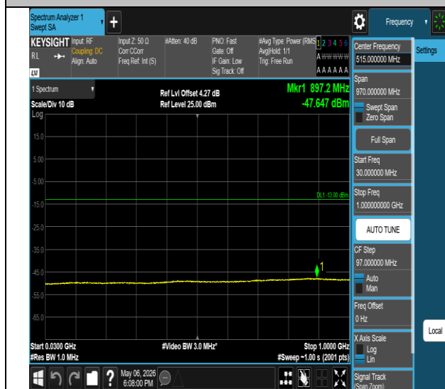
Band IV-1312-30~1000MHz-PASS
