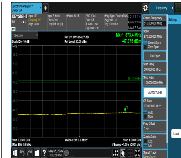
Band II-9400-30~1000MHz-PASS
