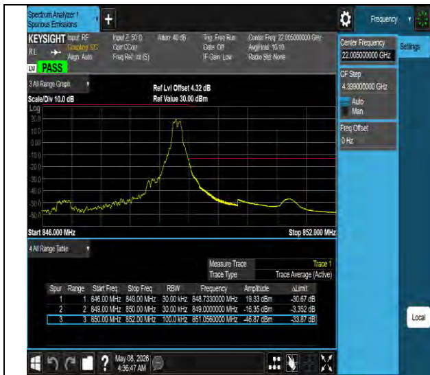
Band26(824-849)-3MHz-QPSK-27025-1RB#14-PASS
