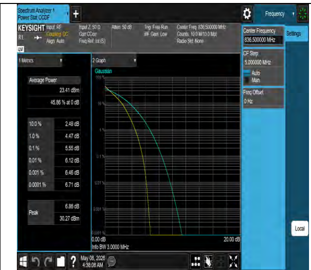
Band26(824-849)-3MHz-QPSK-26915-15RB#0-PASS
