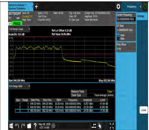
Band26(824-849)-3MHz-QPSK-27025-15RB#0-PASS
