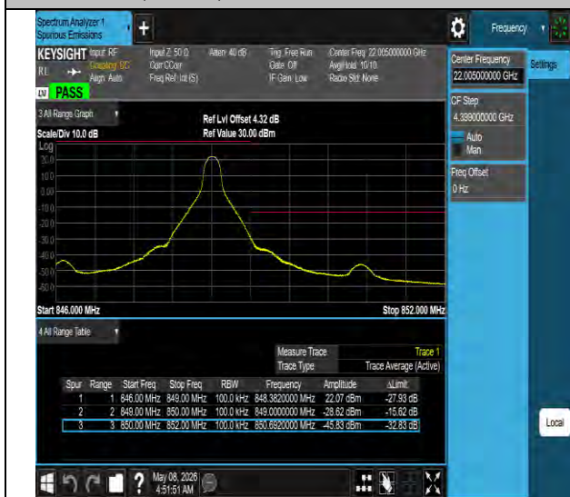
Band26(824-849)-10MHz-QPSK-26990-1RB#49-PASS
