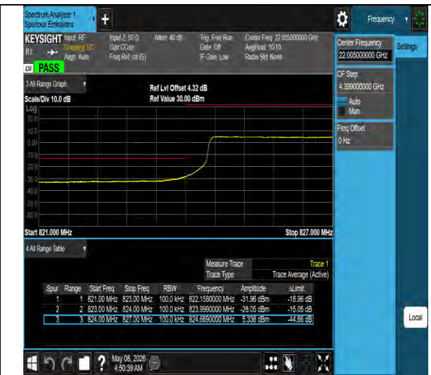
Band26(824-849)-10MHz-QPSK-26840-50RB#0-PASS
