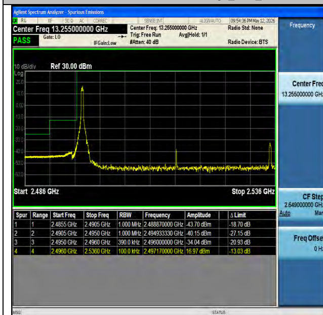
NTNV-n41-PC2-30-40-L-CP-QPSK-Edge_1RB_Left-PASS
