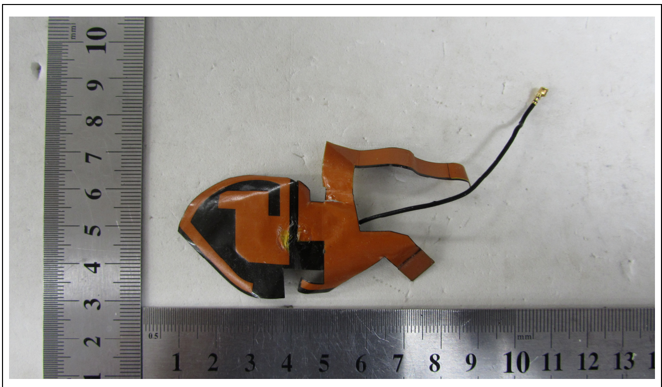
<LTE Antenna>
