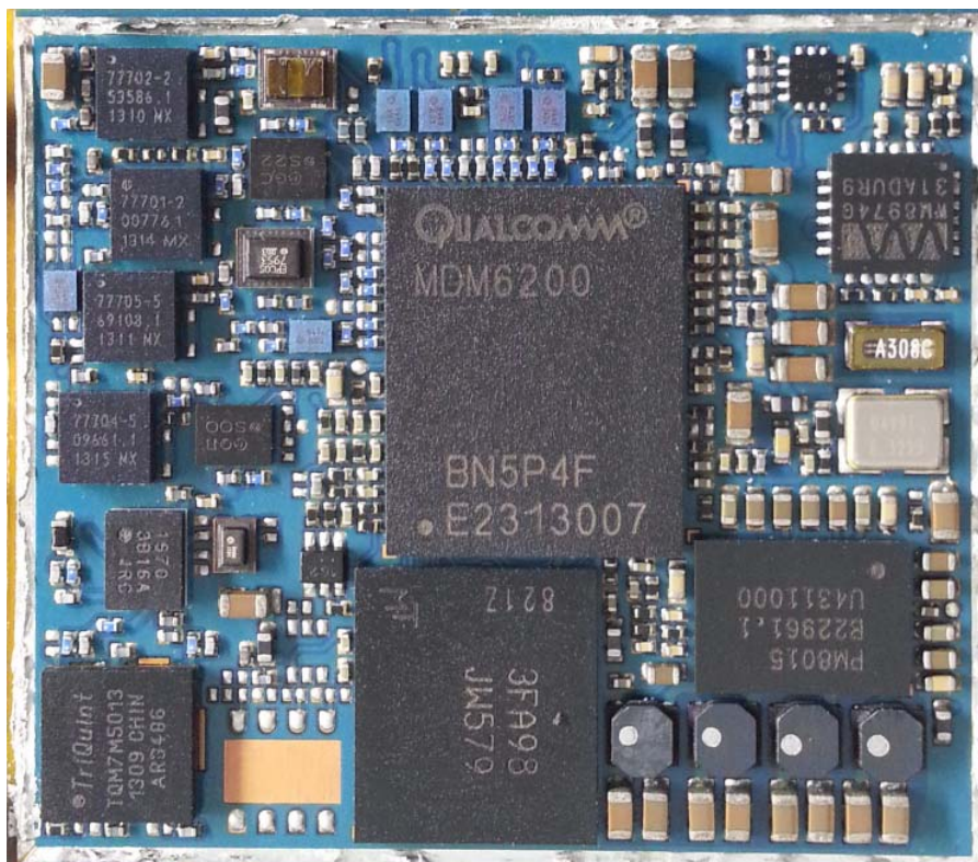
WWAN Module
