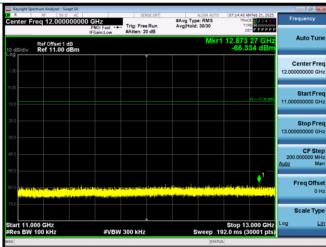
BLE_2M-Ant1-2440-11000~13000-PASS
