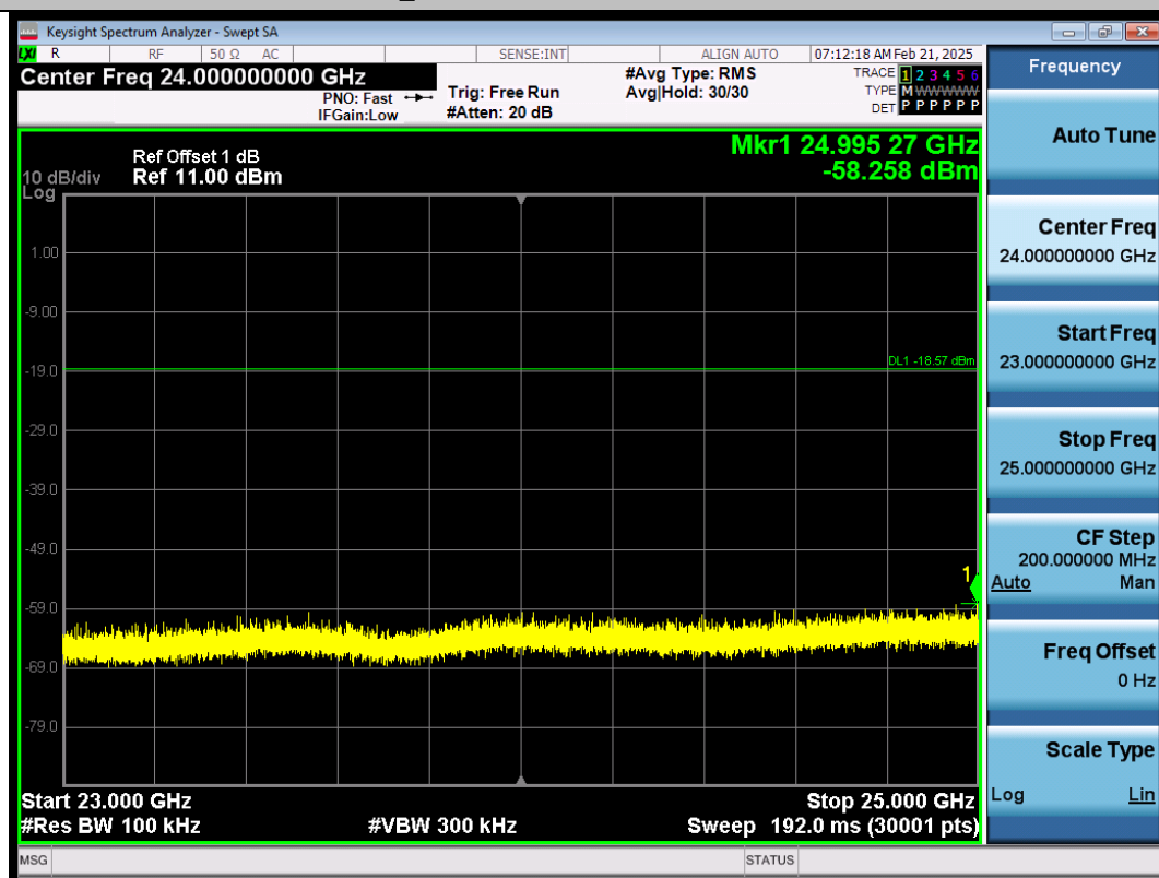
BLE_2M-Ant1-2404-23000~25000-PASS
