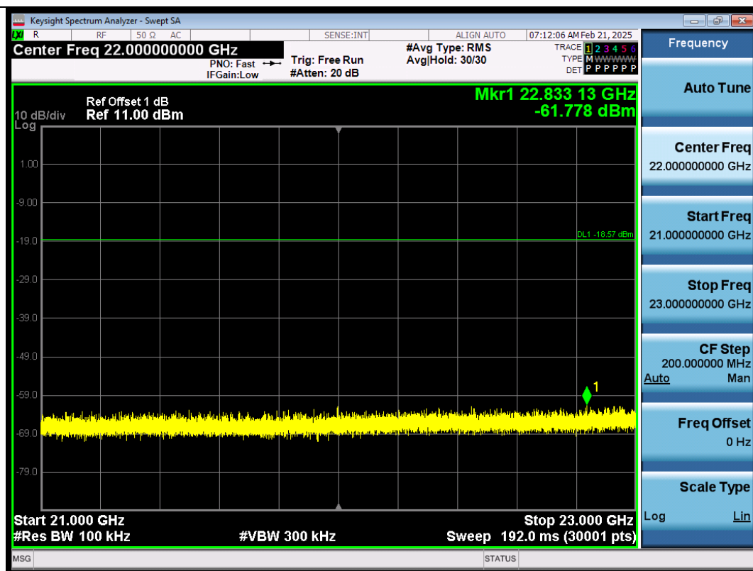
BLE_2M-Ant1-2404-21000~23000-PASS
