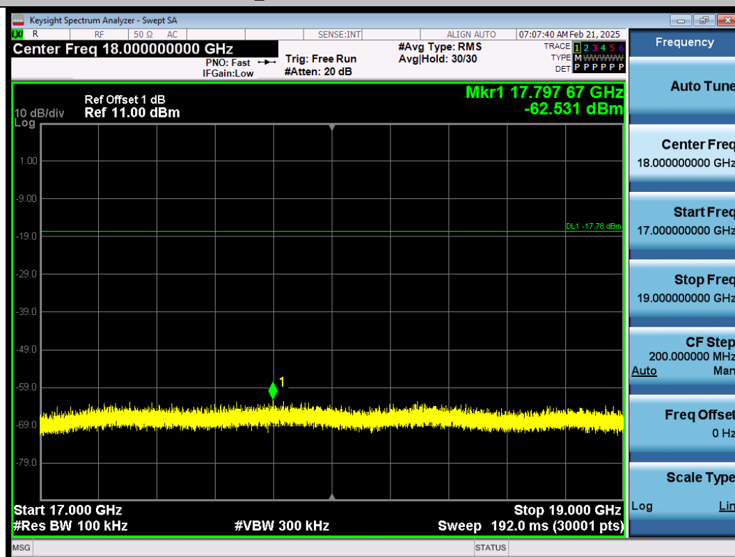
BLE_1M-Ant1-2480-17000~19000-PASS
