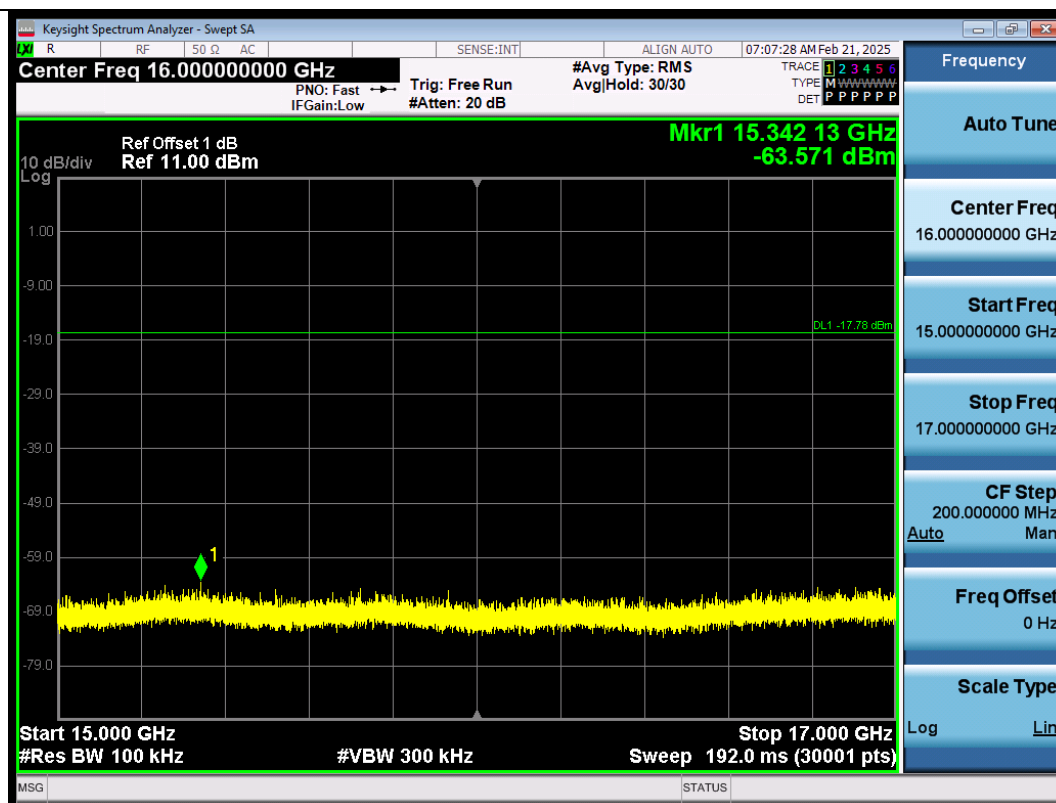
BLE_1M-Ant1-2480-15000~17000-PASS
