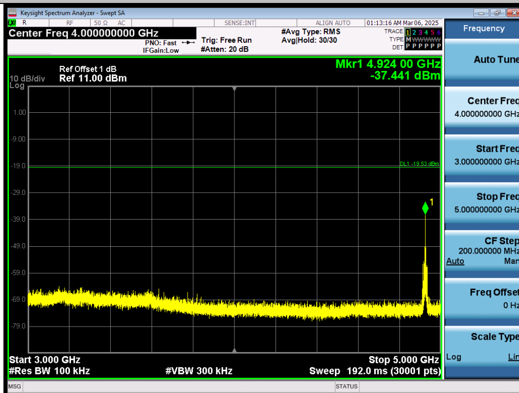
11B-Ant1-2462-3000~5000-PASS
