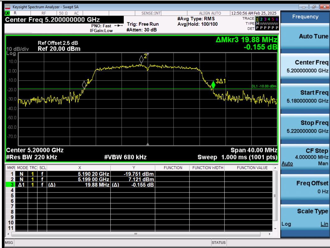
11A-Ant1-5200
