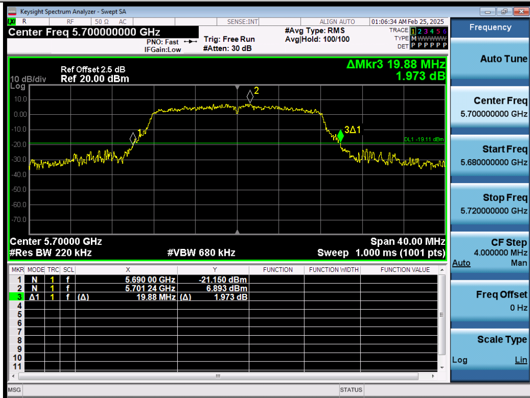
11A-Ant1-5700
