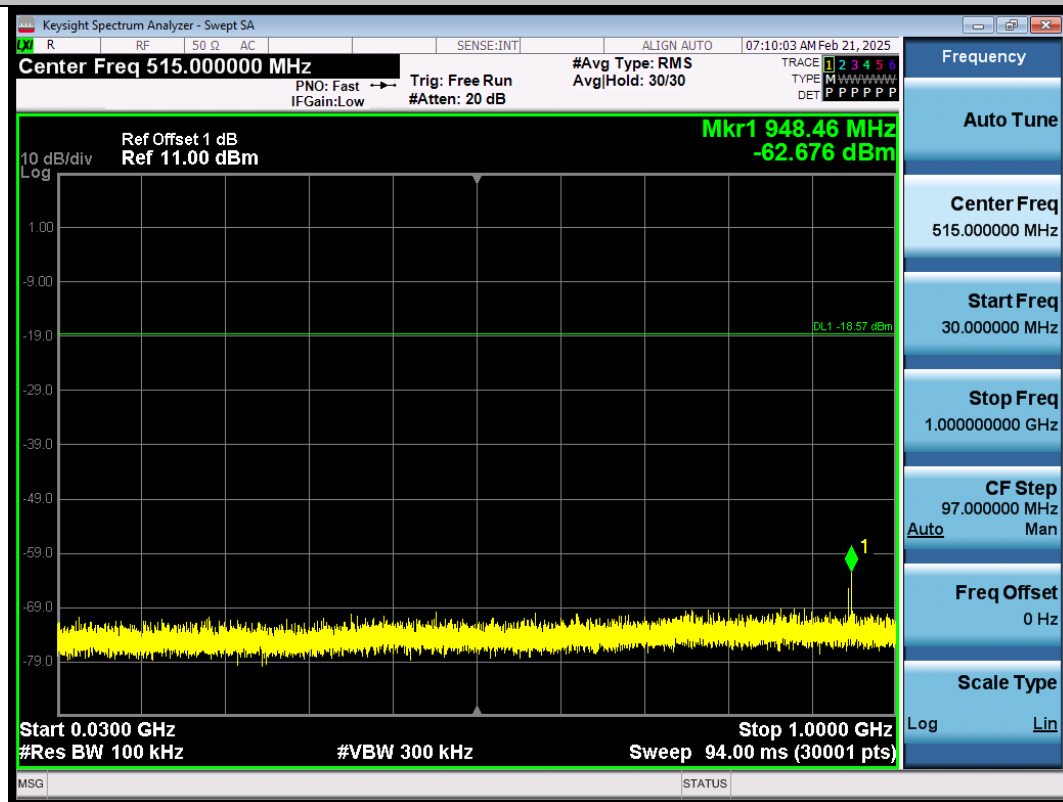
BLE_2M-Ant1-2404-30~1000-PASS
