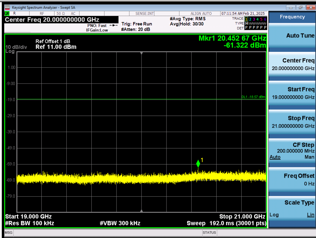
BLE_2M-Ant1-2404-19000~21000-PASS
