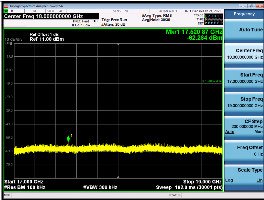
BLE_2M-Ant1-2404-17000~19000-PASS
