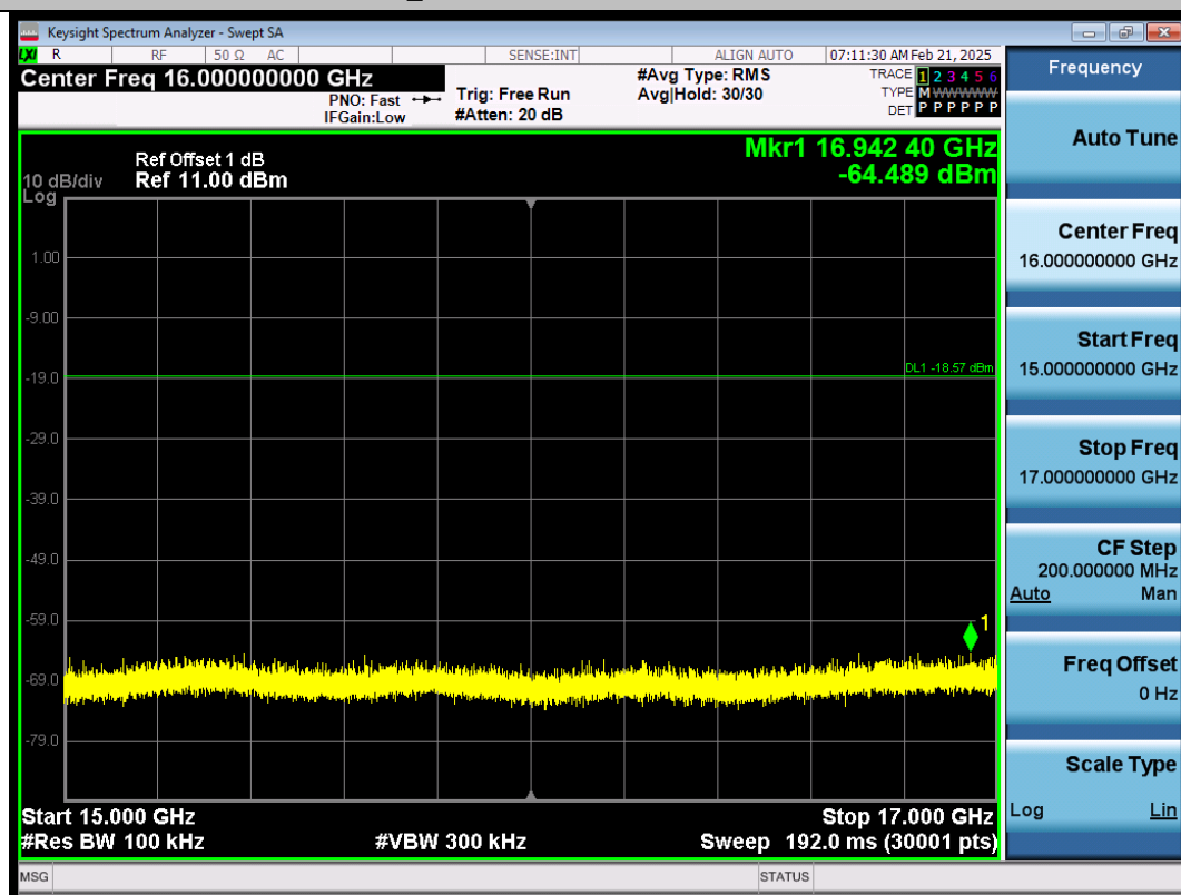
BLE_2M-Ant1-2404-15000~17000-PASS
