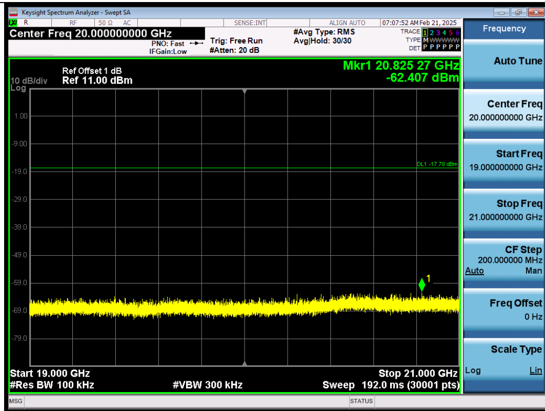
BLE_1M-Ant1-2480-19000~21000-PASS
