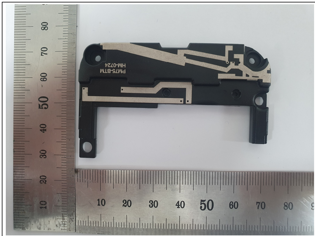
<LTE Antenna>
