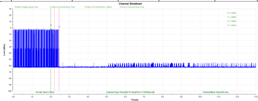
11AC80SISO-5290-Type0-PASS
