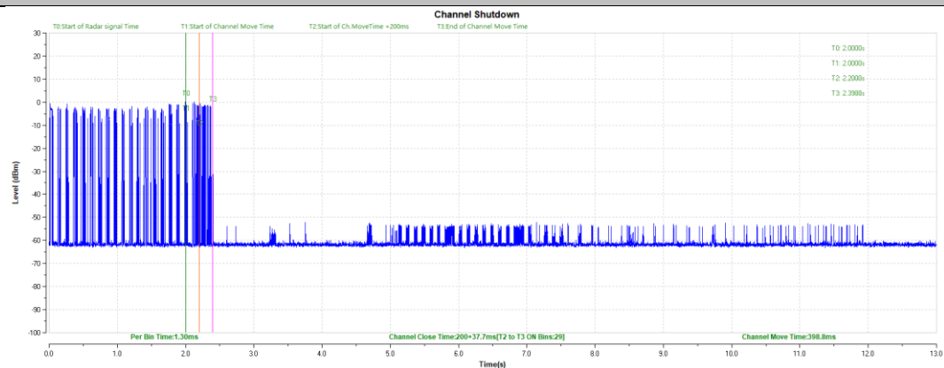
11AC80SISO-5530-Type0-PASS
