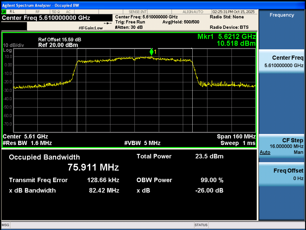
11AC80SISO-Ant3-5610
