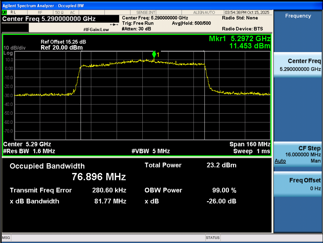
11AX80SISO-Ant3-5290
