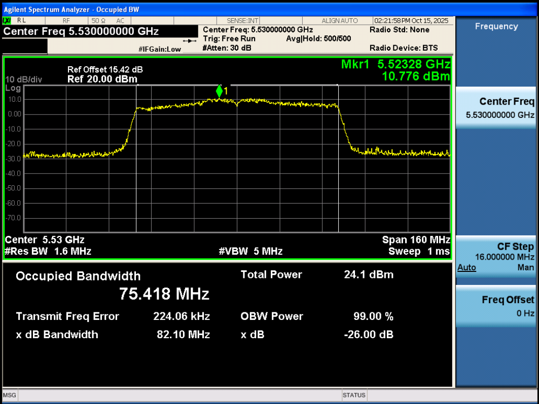
11AC80SISO-Ant3-5530
