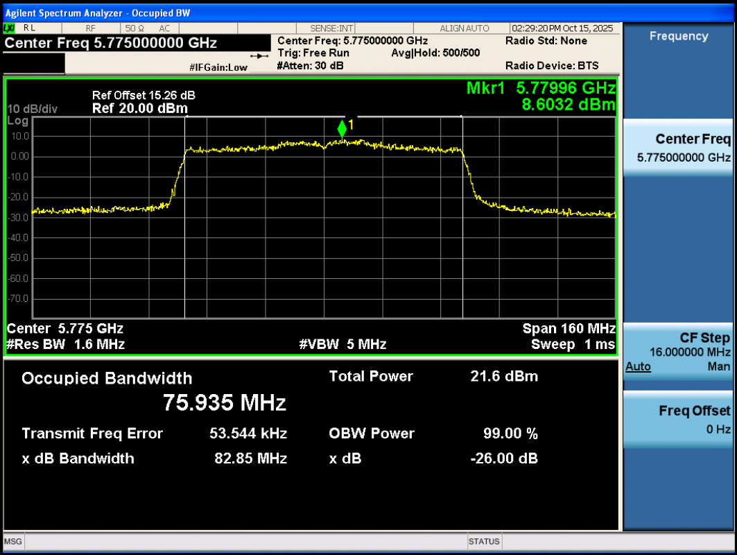
11AC80SISO-Ant3-5775
