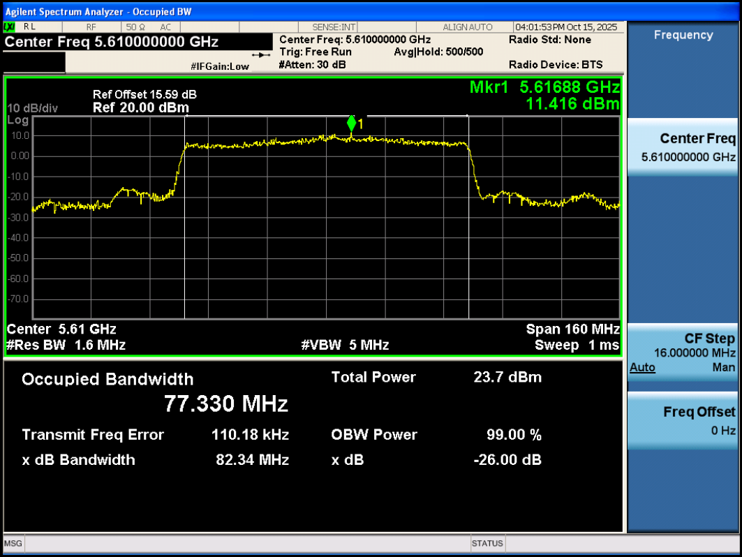
11AX80SISO-Ant3-5610
