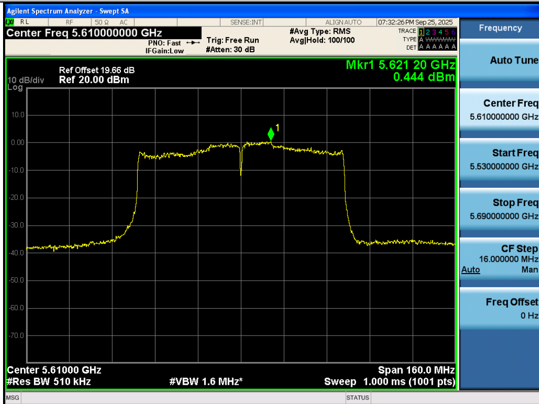
11AC80SISO-Ant3-5610-PASS
