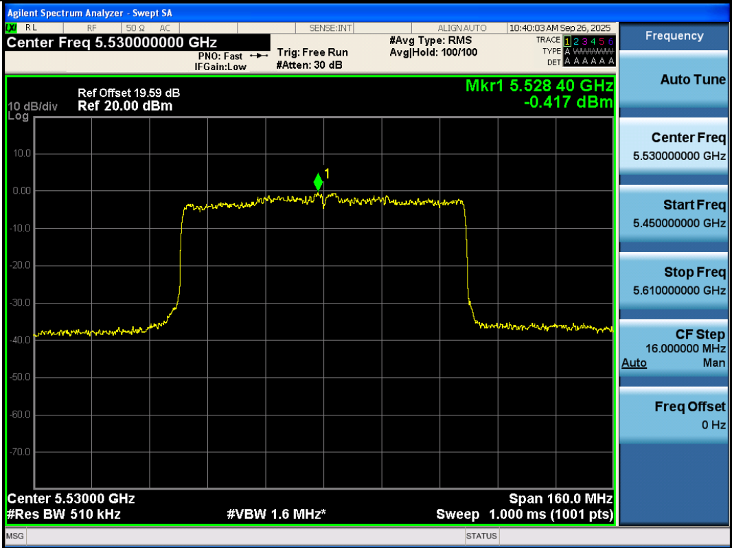
11AX80SISO-Ant3-5530-PASS
