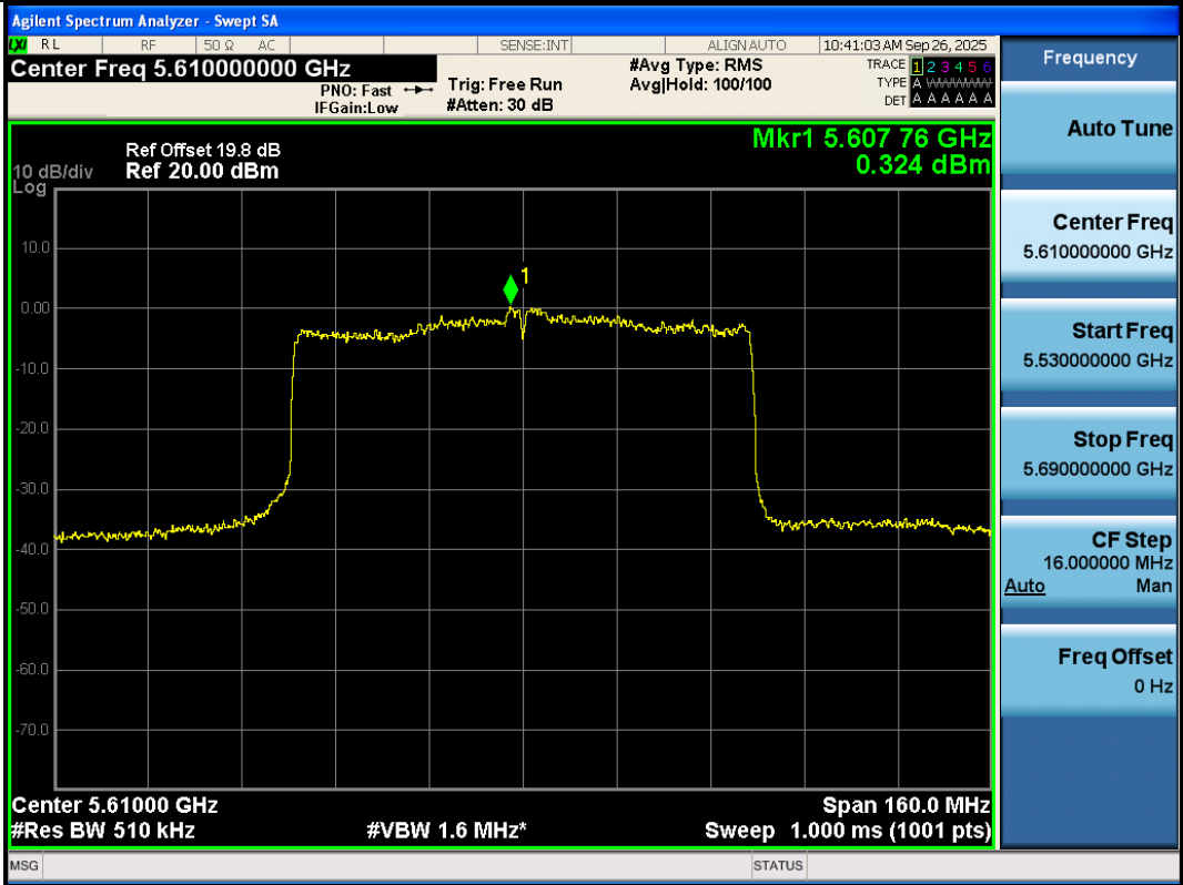
11AX80SISO-Ant3-5610-PASS
