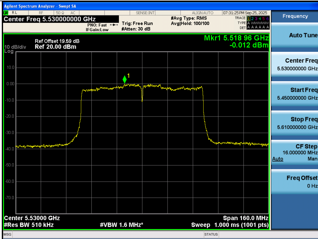
11AC80SISO-Ant3-5530-PASS
