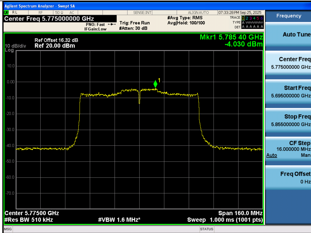
11AC80SISO-Ant3-5775-PASS
