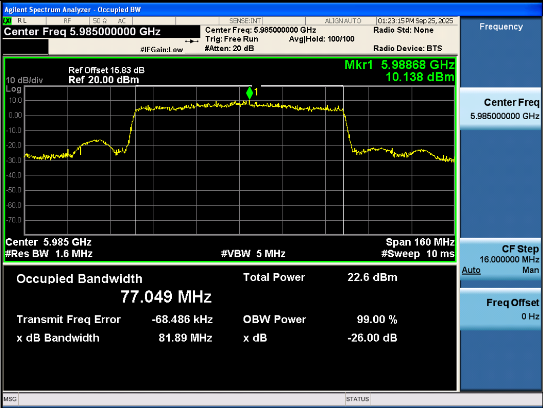
11AX80SISO-Ant3-5985-PASS
