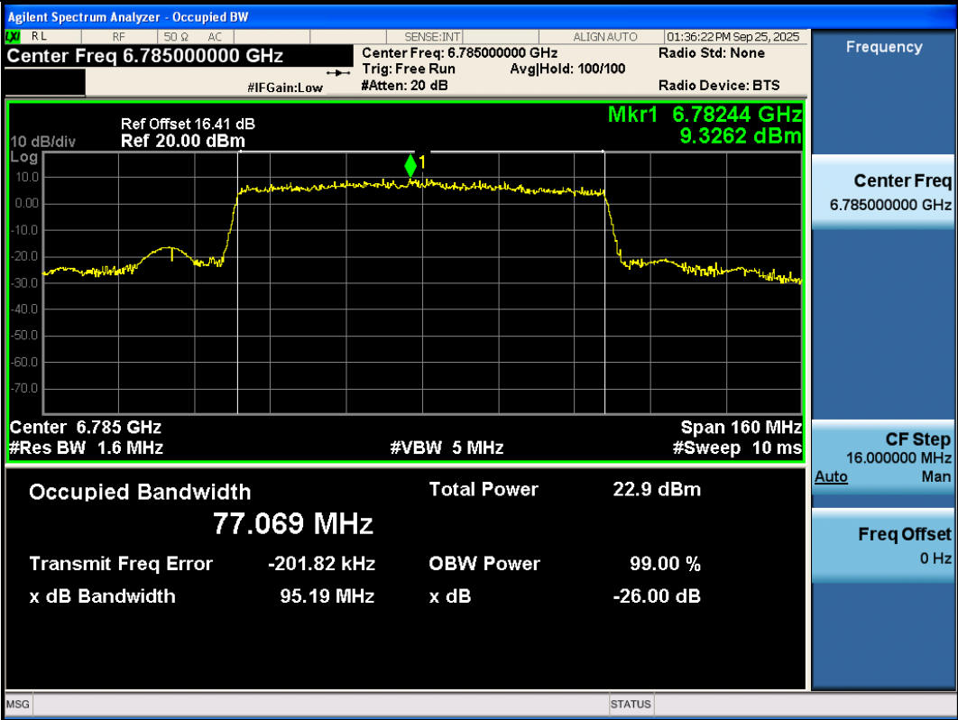
11AX80SISO-Ant3-6785-PASS
