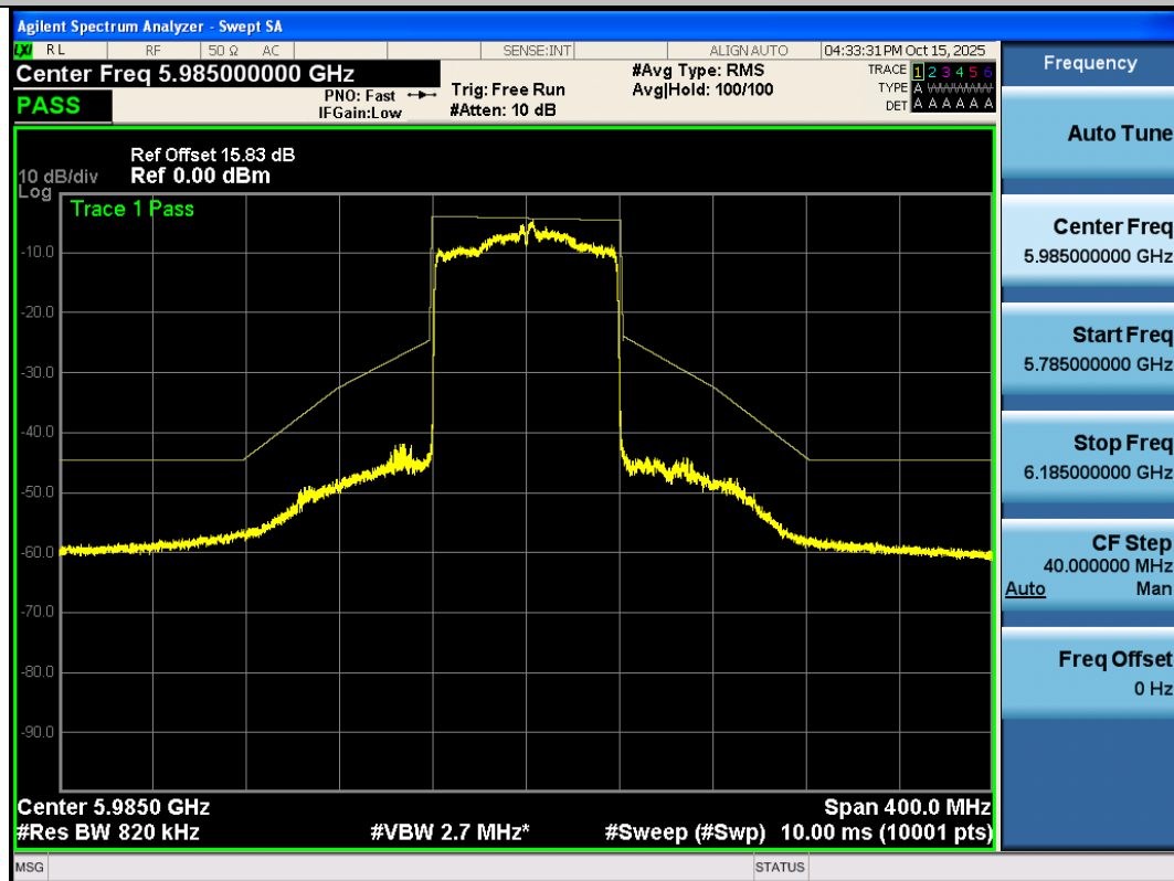
NTNV-11AX80SISO-Ant3-5985-PASS
