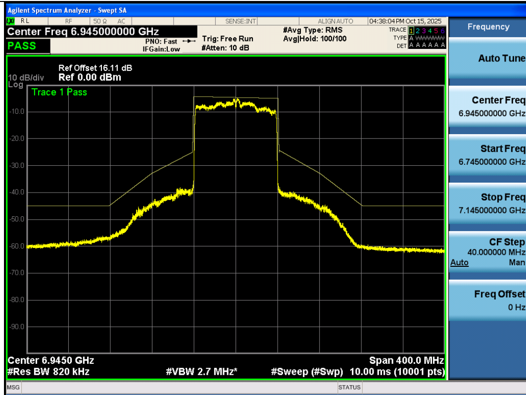
NTNV-11AX80SISO-Ant3-6945-PASS
