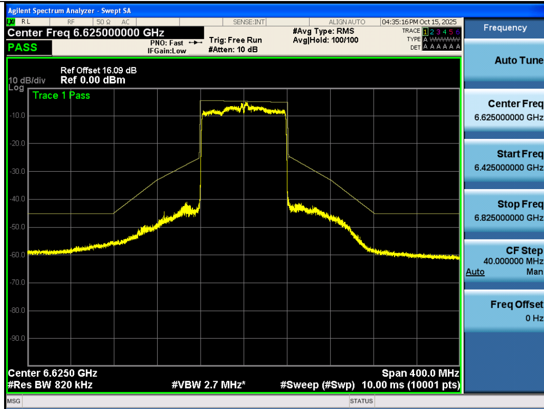
NTNV-11AX80SISO-Ant3-6625-PASS
