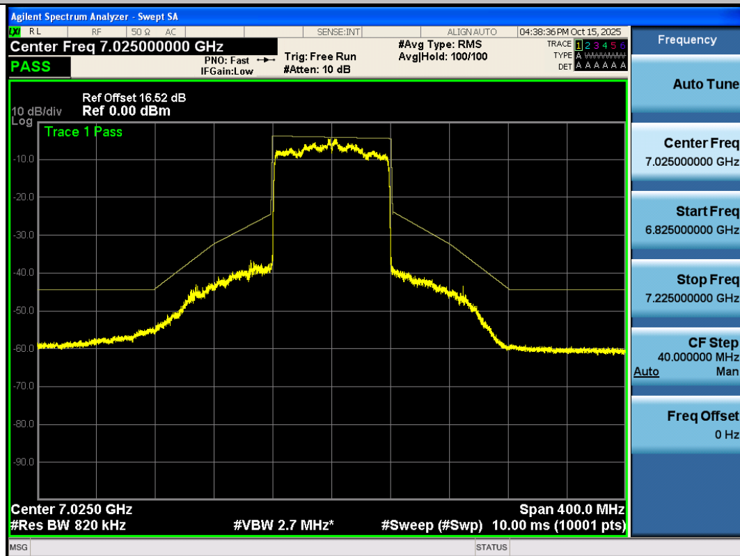
NTNV-11AX80SISO-Ant3-7025-PASS
