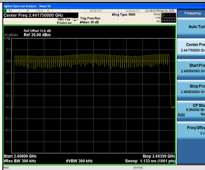
2DH5_Ant2_Hop
