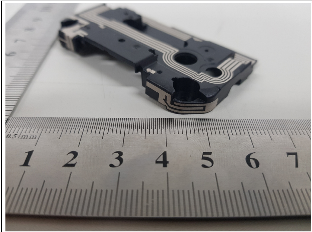
<GPS/WIFI/BT Antenna>
