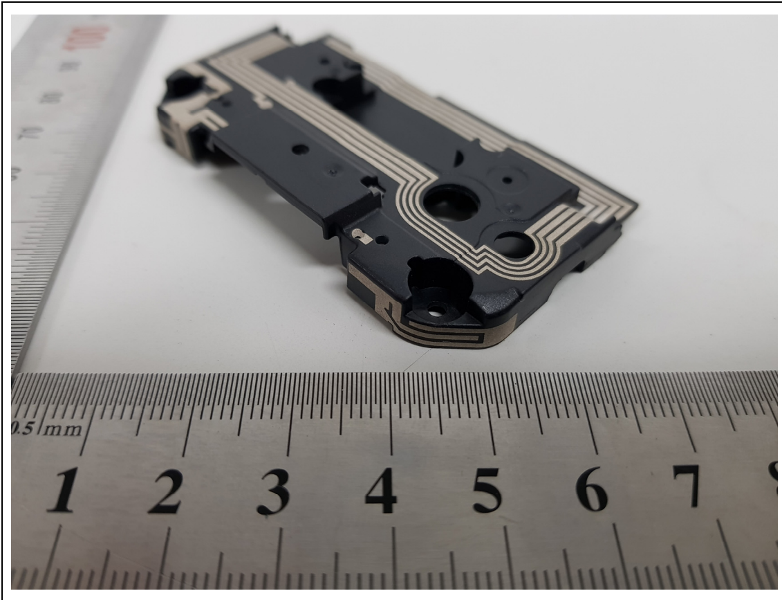
<GPS/WIFI/BT Antenna>
