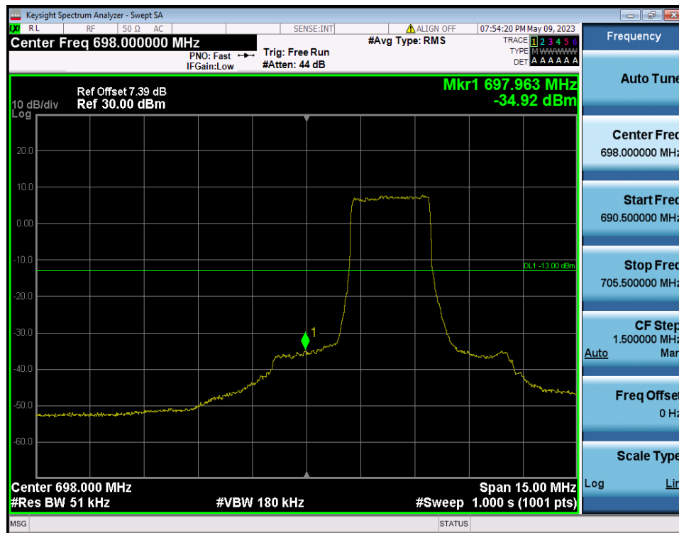
LTE Band 12(17) / 5MHz / QPSK - RB Size/Offset (12/0)
