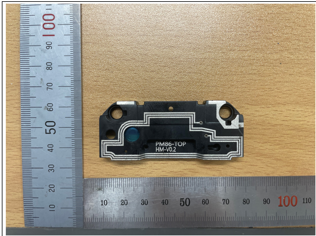
TOP(WLAN, BLE, NFC) Antenna
