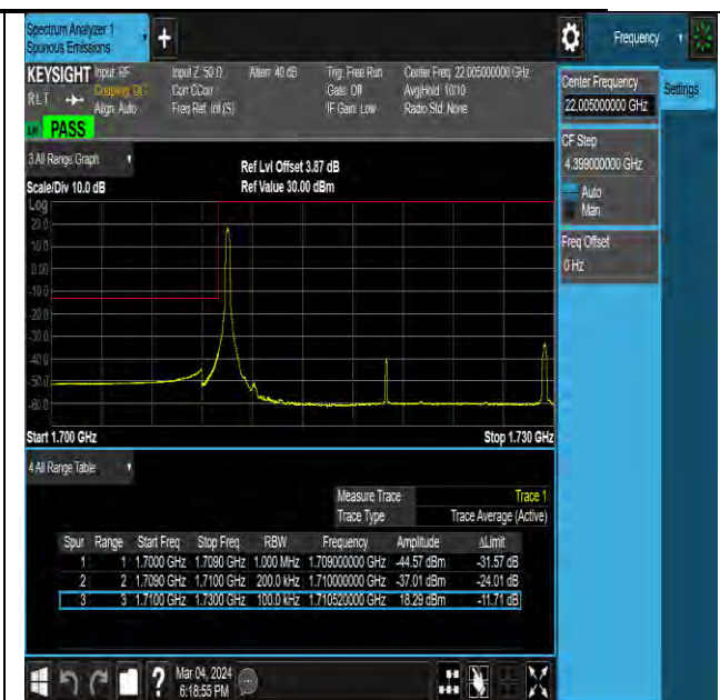
NTNV-N66-PC3-15-20-L-DFT-QPSK-Edge_1RB_Left-Ant1-PASS
