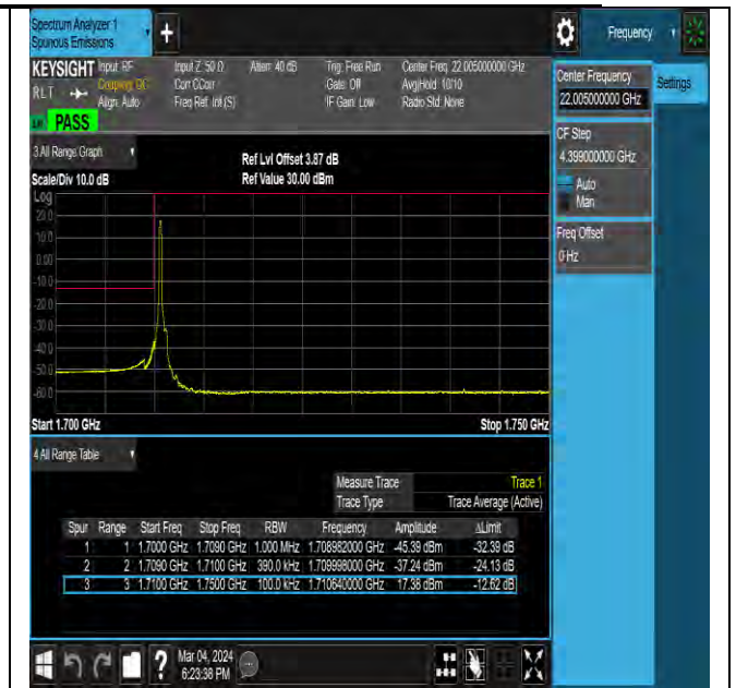
NTVN-N66-PC3-15-40-L-DFT-QPSK-Edge_1RB_Left- Ant1-PASS
