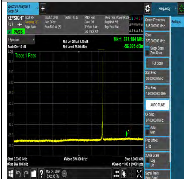
NTNV-N71-PC3-15-10-H-DFT-QPSK-Edge_1RB_Left- Ant0-PASS
