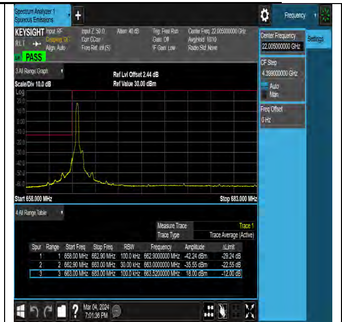
NTNV-N71-PC3-15-20-L-DFT-QPSK-Edge_1RB_Left- Ant0-PASS
