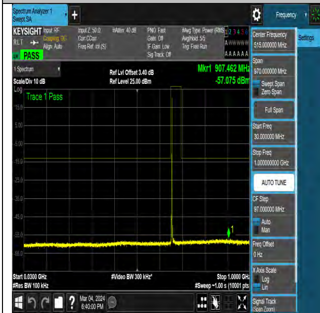
NTV-N71-PC3-15-10-L-DFT-QPSK-Edge_1RB_Left-Ant0- PASS
