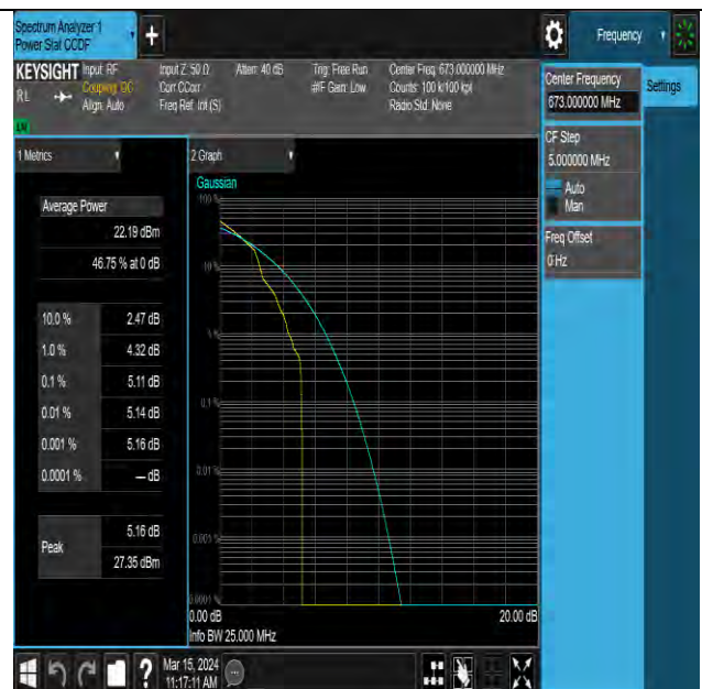
NTNV-N71-PC3-15-20-L-DFT-QPSK-Edge_1RB_Left-PASS
