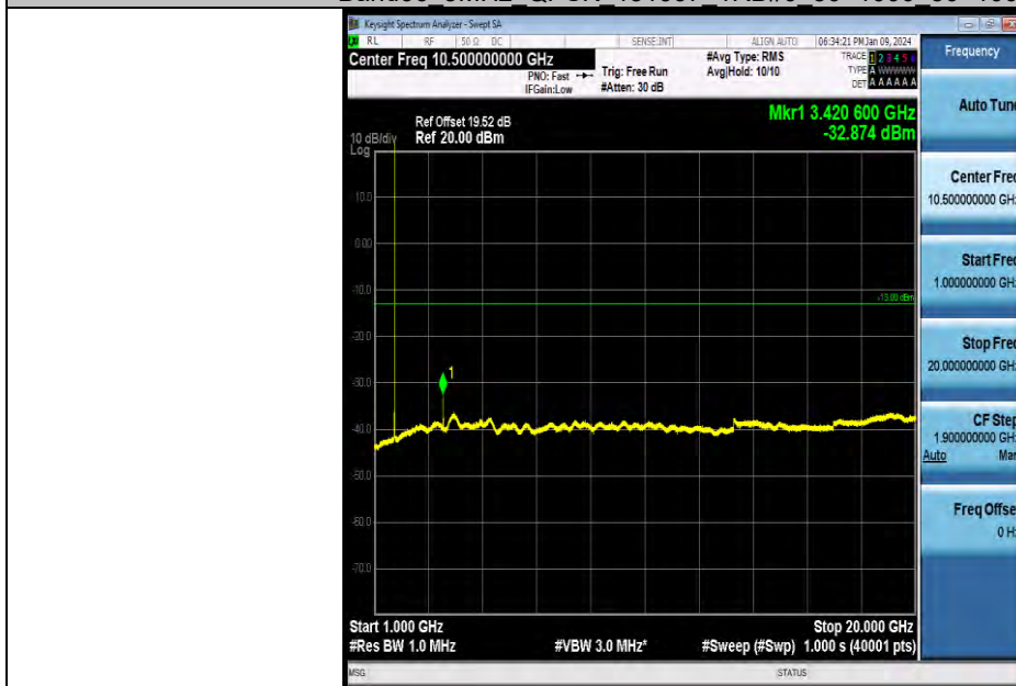
Band66 5MHz QPSK 131997 1RB#0 1000~20000 1000~20000
