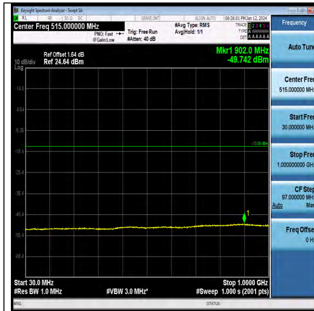
Band4-1513-30~1000MHz-PASS
