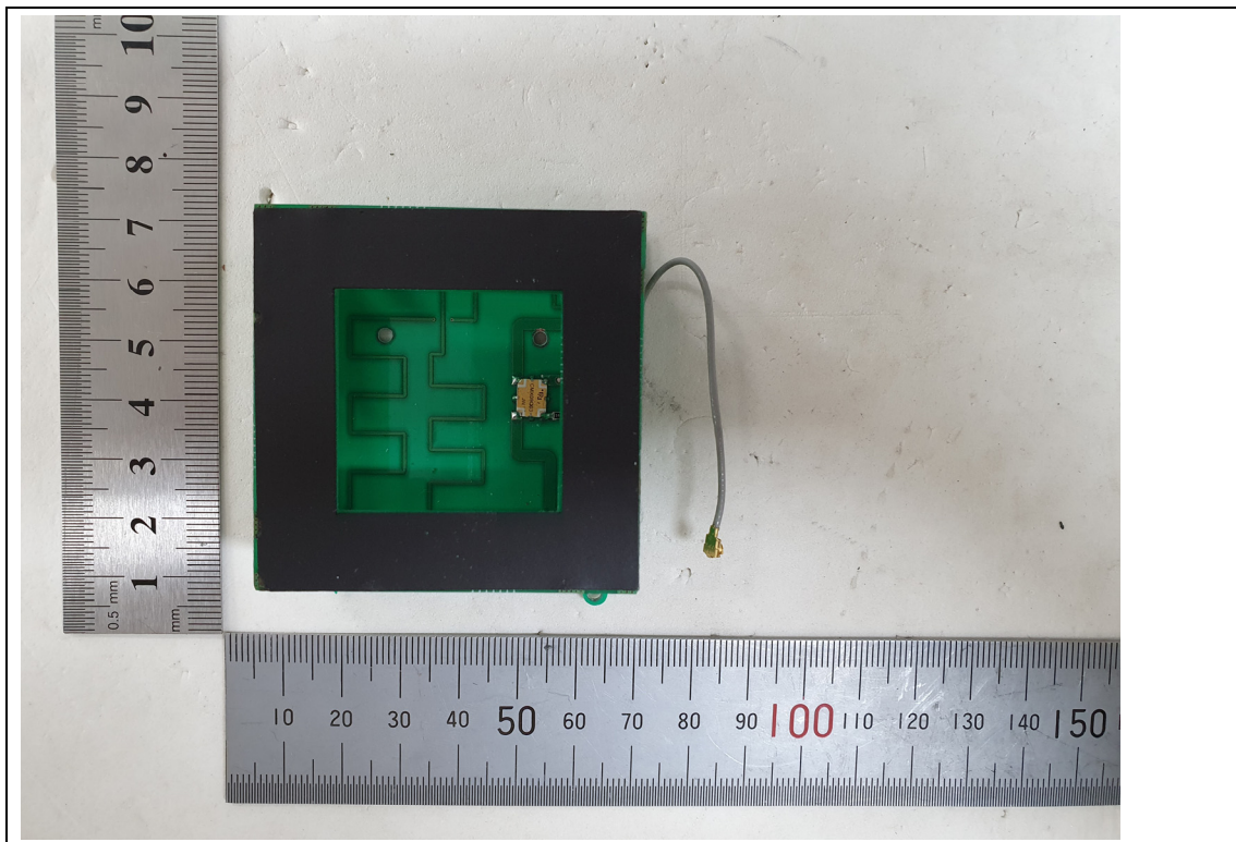
<RFID Antenna>
