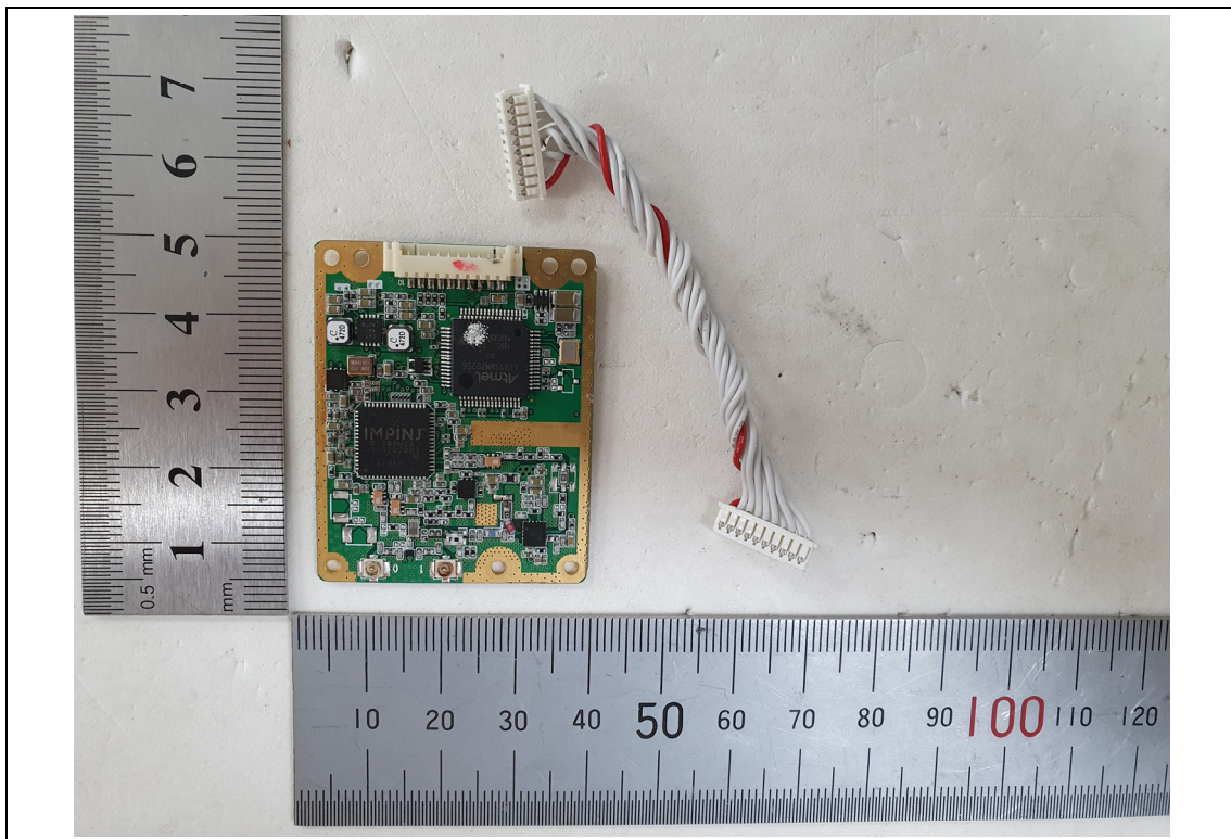
<RFID Module>
