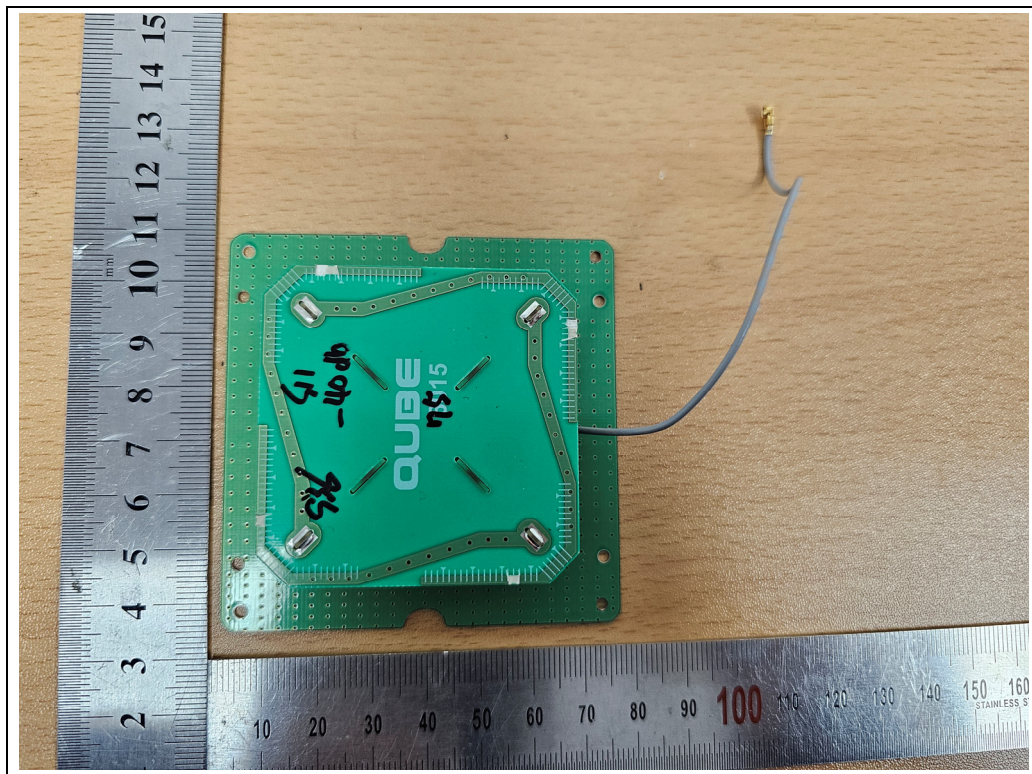
<RFID Antenna>
