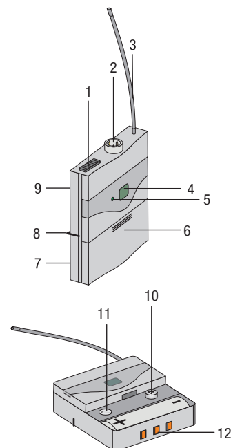
Figura 4: Dispositivos de controlo do transmissor PT420
