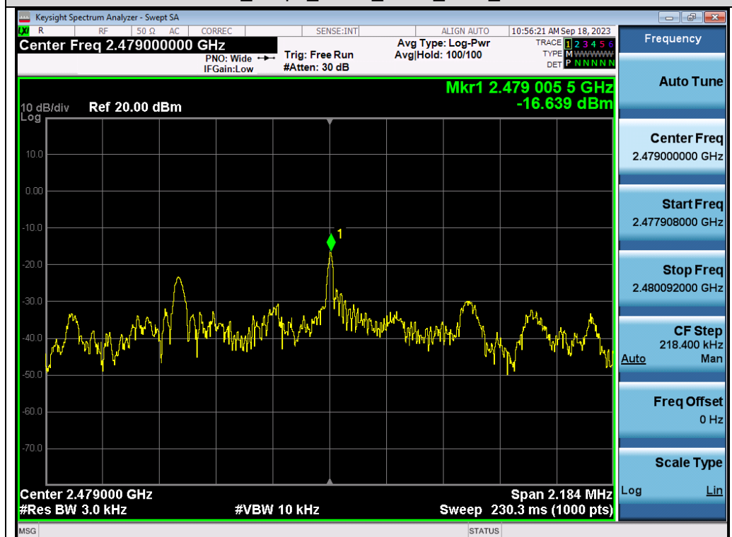
Test_Graph_GFSK_ANT1_2479_PSD
