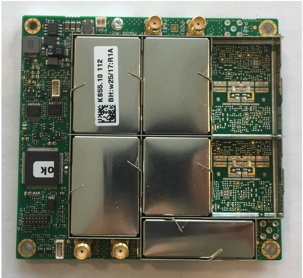
VGA top
