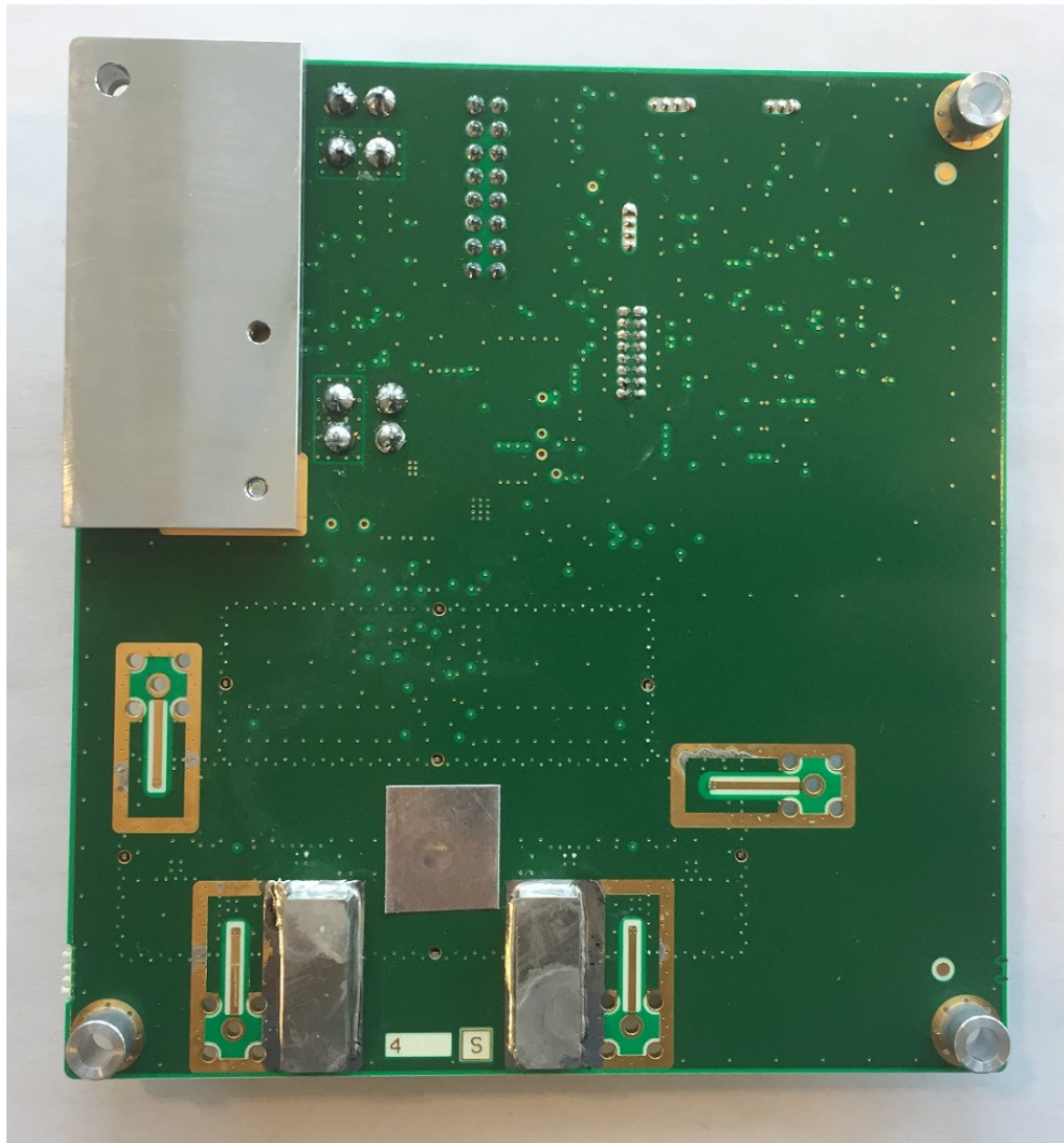
MPI bottom
