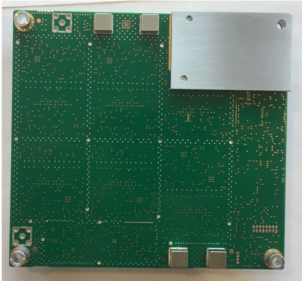
VGA bottom
