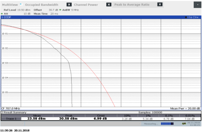
Figure 8.4-8: AGC -0.5 dB 707 MHz PAR UL
