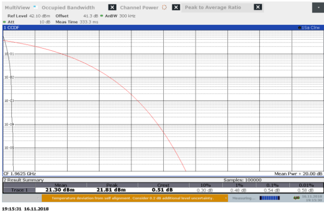
Figure 8.4-8: MSK AGC—0.5 dB 1962.5 MHz PAR DL
