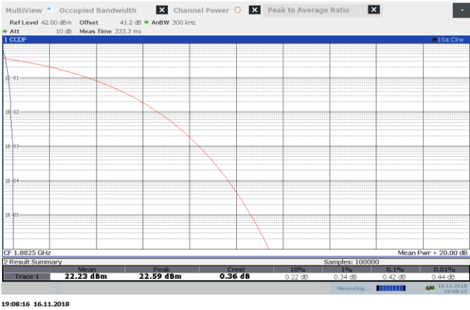
Figure 8.4-12: MSK AGC—0.5 dB 1882.5 MHz PAR UL
