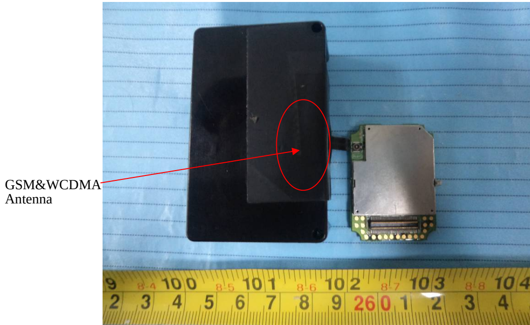
EUT – GSM Module Bottom View
