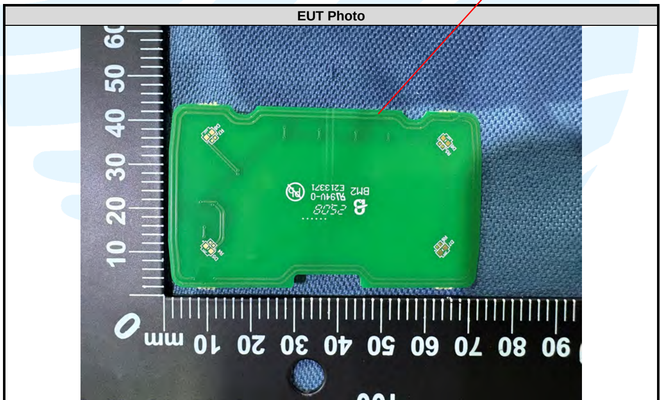
NFC Antenna
