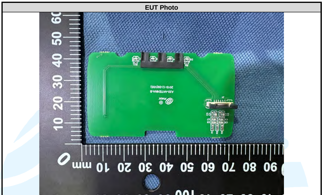
NFC Antenna
