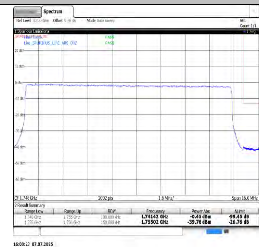
Band4-20MHz-QPSK-20050-1RB#99-PASS
