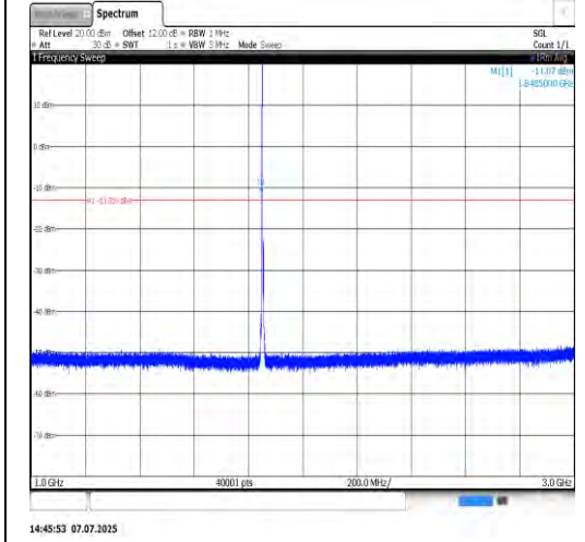
Band2-3MHz-QPSK-18615-1RB#0-1000~3000
